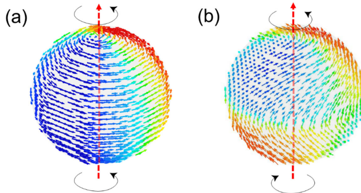
図2: サブミクロン中空球状粒子における(a) 磁気渦、(b)二重磁気渦。 粒子表面のスピン（矢印）の向きを色で表している
