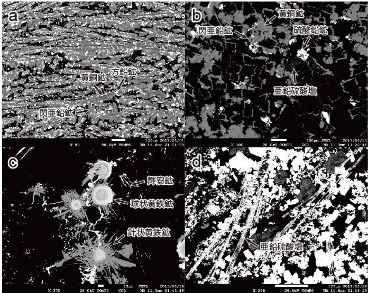
図4 人工熱水噴出孔上に生成したチムニー片の後方散乱電子（BSE）画像。図4a：黄銅鉱と閃亜鉛鉱の樹枝状組織が卓越し、その間を方鉛鉱が埋めている様子、図4b：硫酸塩鉱物が一部溶解あるいは硫化鉱物によって置換されている仮像、図4c：化学累帯構造を示す球状黄鉄鉱、図4d：未同定の重鉛硫酸塩鉱物。
