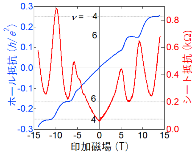
図 2 デルタドーブ SrTiO 3 構造でみられた整数（偶数）量子ホール効果
