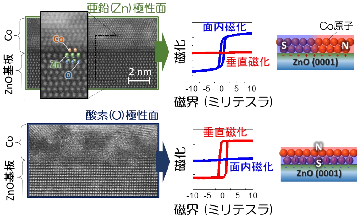
図1：亜鉛及び酸素極性面上に製膜したコバルト薄膜の透過型電子顕微鏡像(左)と磁気特性(中央)。(右)は試料構造と磁化方向を模式的に示したもの。
