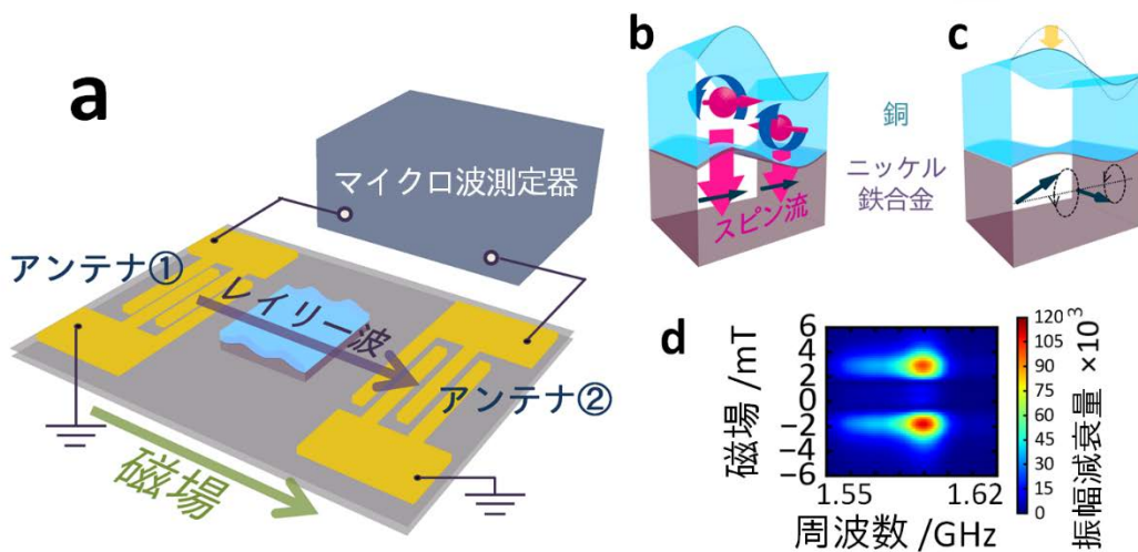
図(a) SAW フィルター素子の構造、(b) レイリー波による交流スピン流生成、(c) 交流スピン流による磁気量の変化とレイリー波振幅の減衰、(d) 磁気量変化の発生によるレイリー波の振幅減衰量
