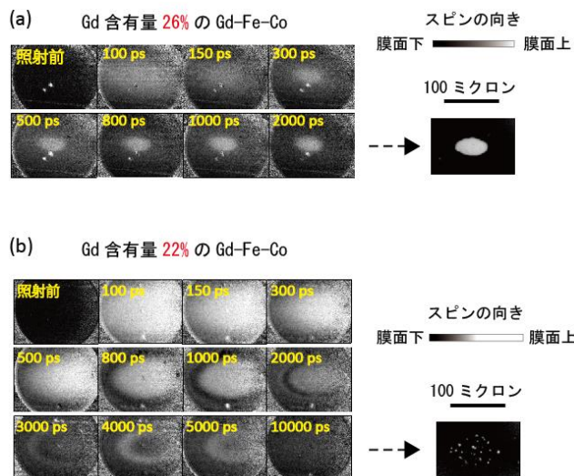
図 4. Gd-Fe-Co 薄膜にレーザーパルス光を照射した直後のスピンの向きを時間経過を示す図。1 ps (1 ピコ秒) は 1 兆分の 1 秒。(a)速やかなスピン反転が期待される Gd 含有量 26%の薄膜では数 100 ピコ秒でスムーズなスピン反転が完了しています。一方、(b)Gd 含有量 22%の試料では、同心円状にスピンの向きが分布した挙動が観測されています。パルス照射から十分な時間が経過した後は ((a)、(b) 各図の右下)、(a)Gd26%試料では綺麗なスピン反転が起きています。一方、(b)Gd22%試料ではほとんどスピン反転が起こらず、大部分の領域で元のスピン方向に戻っています。
