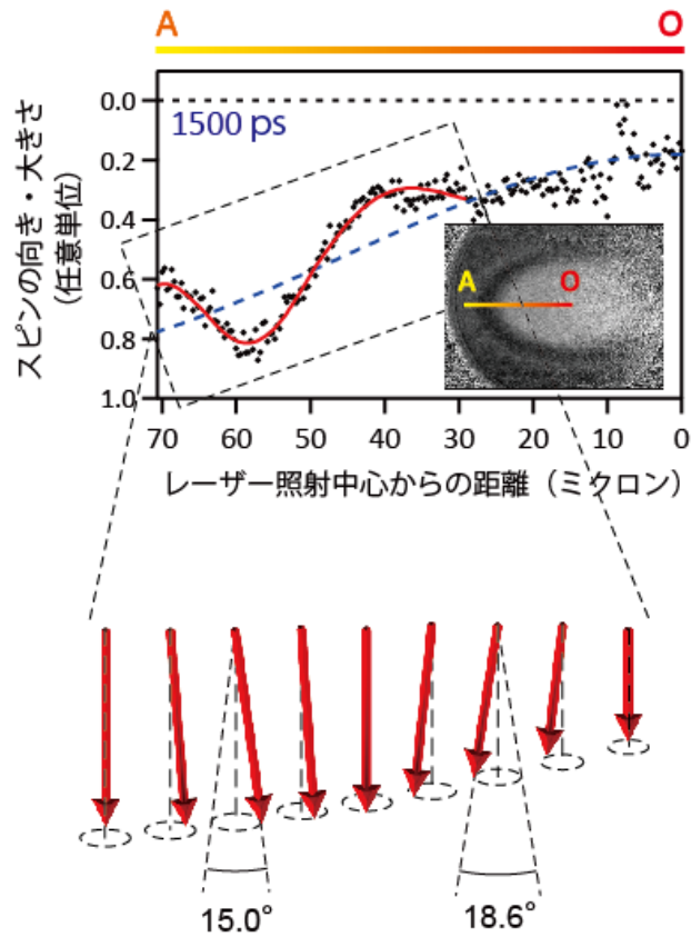
図5. Gd22%含有のGd-Fe-Co薄膜におけるレーザーパルス光照射後1500ピコ秒でのスピンの分布。上部図の挿入画像が得られた磁気像、上部プロットがレーザー照射中心から半径方向(O-A)の磁気シグナルのラインプロファイル、下部図がラインプロファイルを基に算出したスピンの向きの分布を示しています。歳差運動角約15~20°の伝搬スピン波が生成されていることが分かります。
