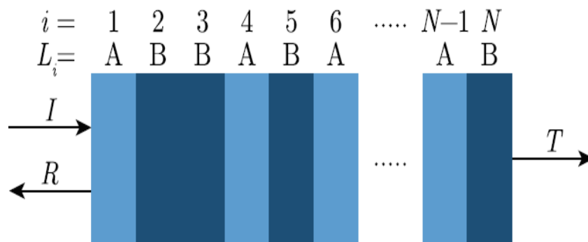
図 1. ランダムに N 枚並べた A と B の 2 種類の誘電体多層膜への電磁波の入射、透過、反射の概念図。 i は膜のラベル、 L_i は膜の種類（A か B）、 I は入射する電磁波、 T は透過確率、 R は反射確率を示す。 2 の N 乗通りのすべての構造を計算すると、透過確率が取り得る値の種類は (N/2+1) 通りしかなかった。
