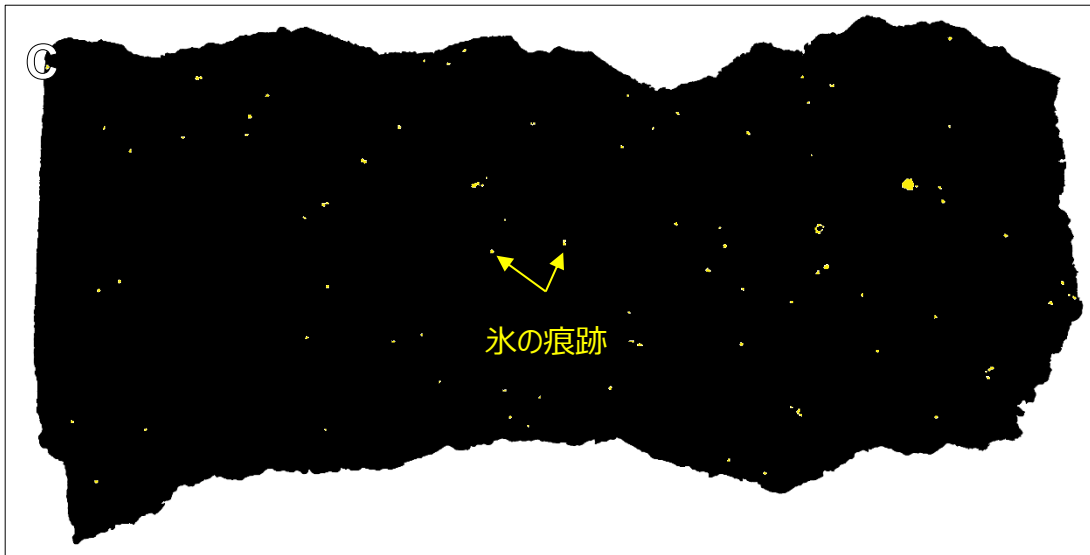
図 3 : (A) 氷の痕跡の電子顕微鏡写真、暗い灰色の空隙が多く見られる。 (B) Acfer 094 隕石試料の広範囲の電子顕微鏡写真と (C) 試料内の氷の痕跡の分布の様子。氷の痕跡は、隕石内に万遍なく見られる。Copyright: Megumi Matsumoto et al.
