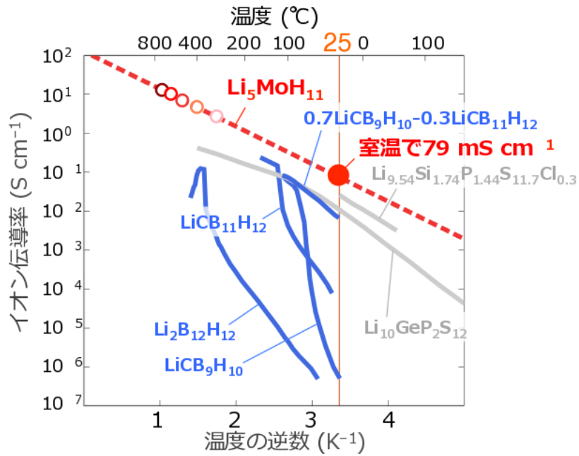
図 3. Li 5 MoH 11 (赤線) および既知の物質におけるイオン伝導率の温度依存性。本研究で見出した Li 5 MoH 11 は、これまでに報告されているどの物質よりも優れたイオン伝導性を示し、室温におけるイオン伝導率は、従来の世界記録を 3 倍以上も更新する 79 mS cm -1 に到達します。
