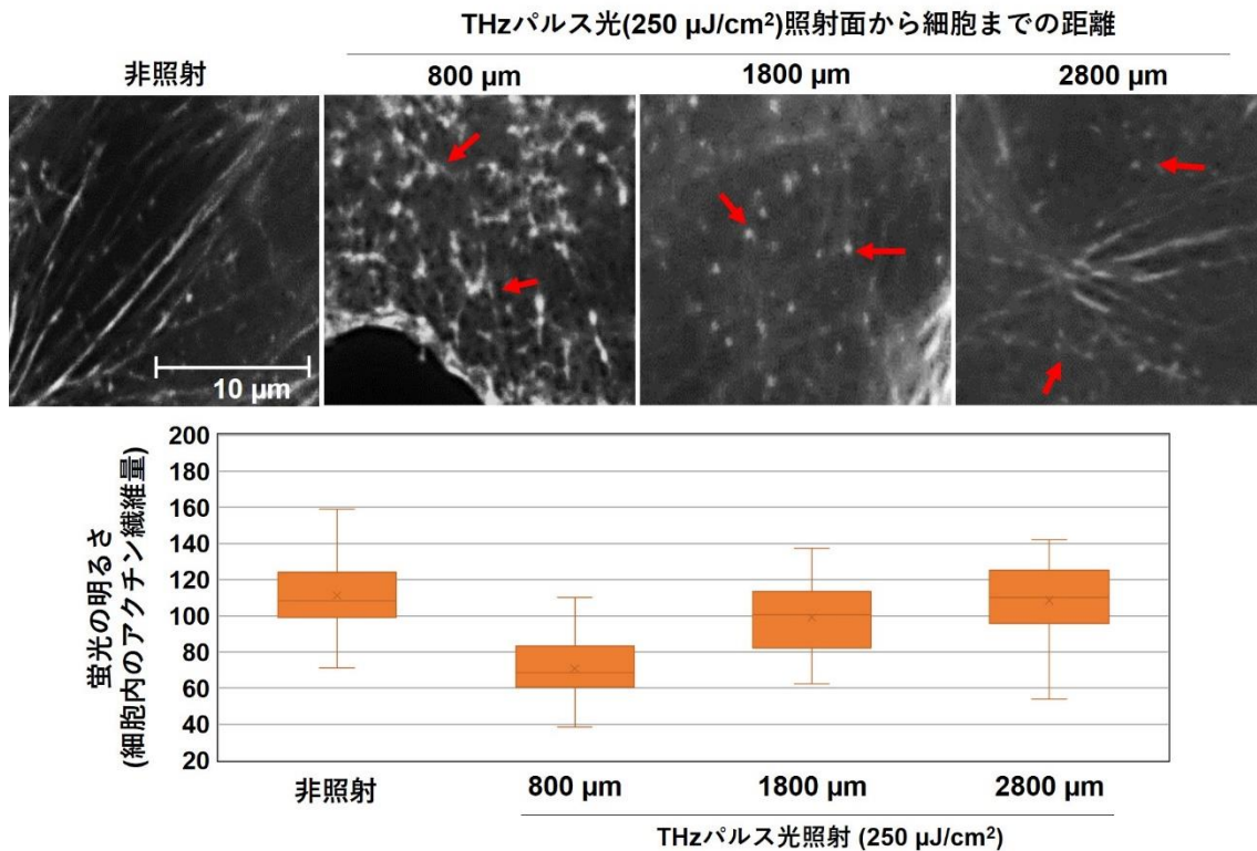
図 2 THz パルス光の照射による細胞内アクチン繊維への影響
