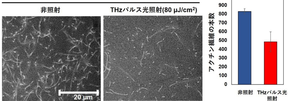
図 1 THz パルス光の照射によるアクチン繊維形成への影響
