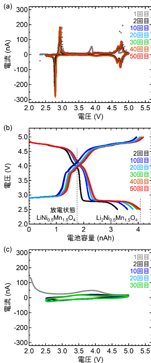
図1 \text{LiNi}_{0.5}\text{Mn}_{1.5}\text{O}_4 全固体電池の充放電測定の結果
