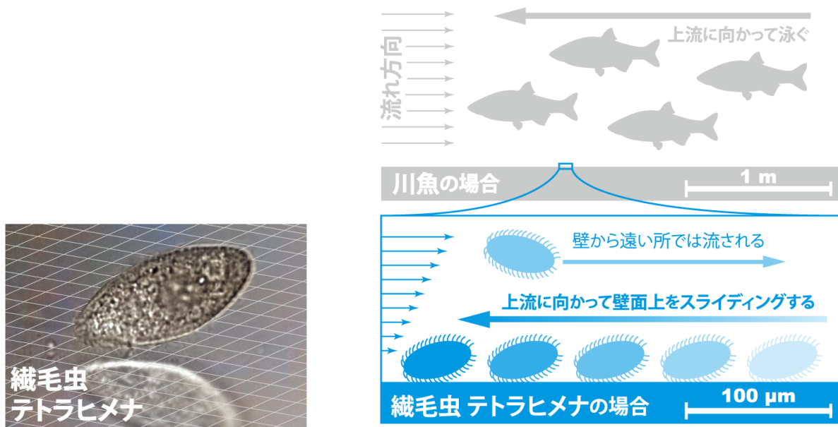
図1. テトラヒメナの顕微鏡写真(ガラス面を識別できるように画像加工)。本研究の模式図(右)。
