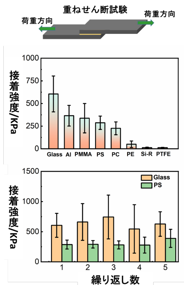
図 2 各材料表面への接着力(上) 繰り返し特性(下)
