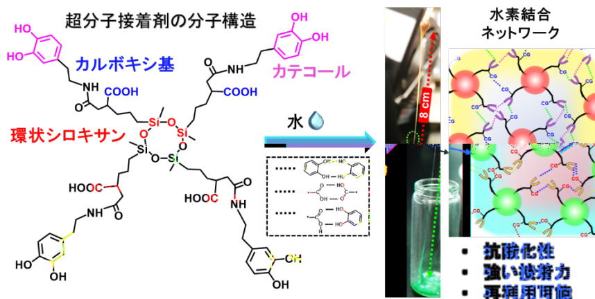
図1 今回開発した超分子接着剤の分子構造。1つの環状シロキサンに4つのカテコール基とカルボキシ基が導入されている。水添加により分子間で可逆的な水素結合のネットワークが形成される結果、抗酸化性や再利用可能といった接着特性があらわれる。
