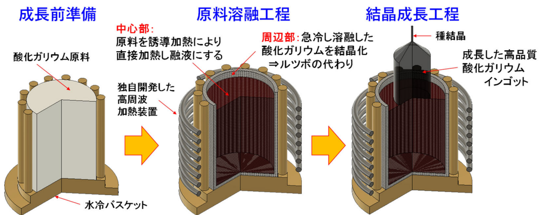
図 1:開発した新規成長法: Oxide Crystal growth from Cold Crucible (OCCC) method
