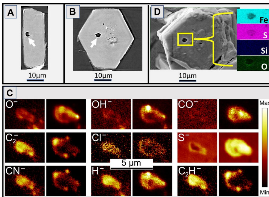
図 5: リュウグウサンプル中の六角板状の結晶(硫化鉄)の内部に発見された水とCO 2 を主成分とする液体。(A、B)硫化鉄結晶中の空孔の CT 像。数ミクロンの大きさの空孔(白矢印)が結晶中に存在している、(C)質量分析計で測定した空孔内に含まれていた様々なイオン種(同じ分子種の2枚の写真は、左側が空孔上部、右側が空孔中部に含まれていたイオン種を示す)。結晶の温度を-120℃にして、空孔中の液体を凍らせて分析した。(D)分析後の空孔中の液体を蒸発させて、空孔内部を観察した結果、結晶を構成する元素(鉄と硫黄)以外は検出されなかった。空孔内には液体以外の固体成分は存在しないことを示す。
