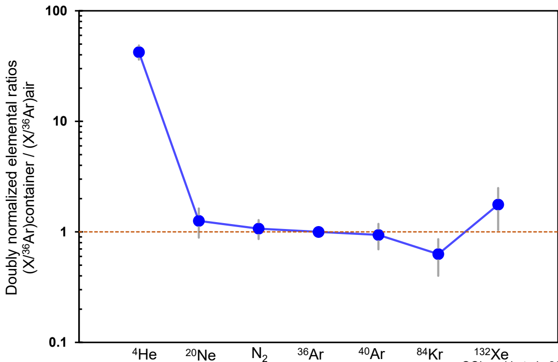
図 3: コンテナガスの元素存在度 (青実線)。測定誤差は灰色棒で示している。縦軸は 36 Ar と地球大気組成で規格化した存在度。横軸はガス種を示す。ヘリウムは地球大気 (オレンジ色点線) に比べてひと桁以上過剰である。
