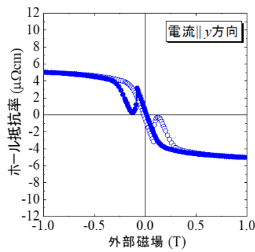
図2 本実験で得られた通常のホール効果と異方的なホール効果の対比
