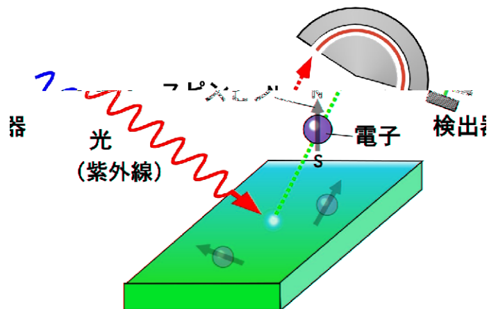
図 3: スピン分解光電子分光法. 紫外線の照射によって物質外に放出された電子のエネルギー・運動量・スピンを観測する.
