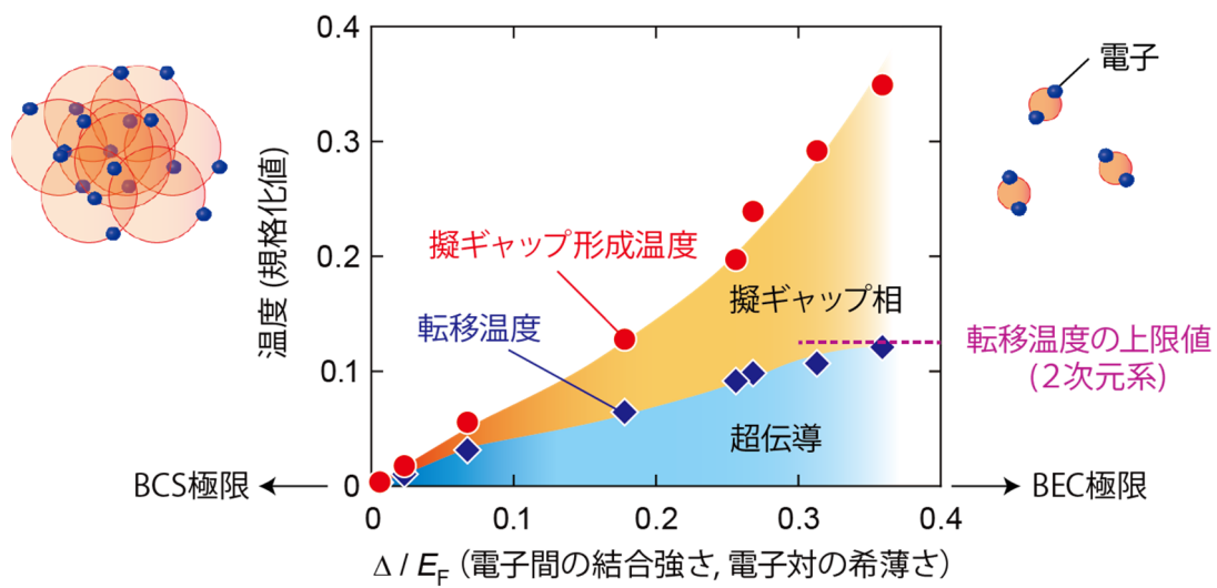
図3. 本研究で得られた ZrNCl の超伝導相図。縦軸は電子の運動エネルギーで規格化された温度、横軸は電子間の結合の相対的な強さ、すなわち電子対の希薄さを表すパラメータである。電子対の重なりが小さくなった BCS-BEC クロスオーバー領域で、転移温度の上限値（紫破線）に到達している。枠外の図は BCS 極限、BEC 極限における電子対の模式図。
