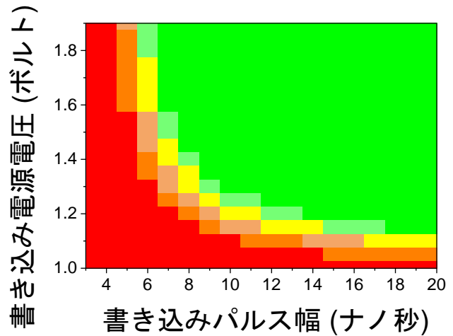
図2 アドバンテスト社製メモリテストシステムを用いて評価した 128Mb 密度の STT-MRAM 内のサブアレイの高速動作特性評価の結果。
