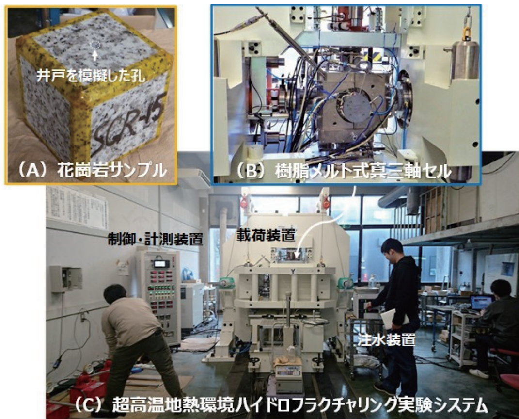
図 1: 超高温地熱環境ハイドロフラクチャリング実験システムと実験風景。本実験システムは、立方体状の岩石サンプル(写真 A)を格納する樹脂メルト式真三軸セルと呼ばれる特殊な高温対応耐圧容器(写真 B)と、このセルとともに使用して岩石の加熱加圧を行う载荷装置や制御・計測装置,そして岩石に注水するための注水装置などから構成されています(写真 C)。
