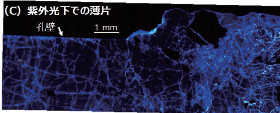
図 2:450°Cでのハイドロフラクチャリング実験後の花崗岩サンプル内に形成された高密度に分布する微小き裂からなる透水性き裂ネットワーク。実験後の花崗岩サンプルの上面にある孔から水を注入すると、他の面から多数の水滴が出現し(写真 A)、サンプル内部に透水性き裂ネットワークが形成されていることがわかったため、サンプルに紫外光照射下で青白く蛍光する樹脂を含浸させた後、サンプル内部の薄片を作成して観察した結果(写真 B および C)、高密度に分布する微小き裂からなる透水性き裂ネットワークの形成を確認しました(写真 C の青白い部分が透水性き裂)。
